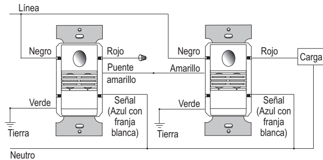
Cableado en dos fases
