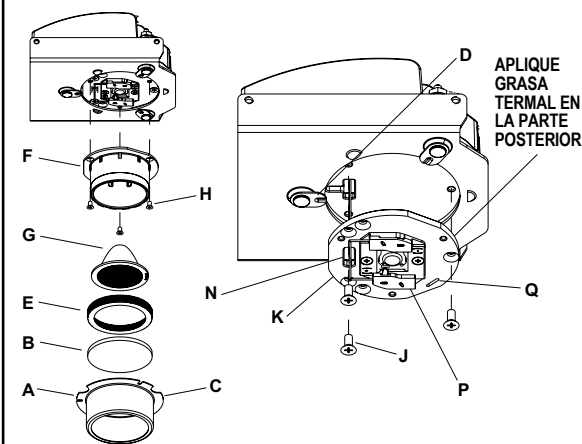
Fig. 11b: Carcasa destinada a bañador de pared
