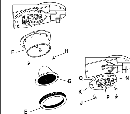
Fig. 11b: Carcasa destinada a bañador de pared
