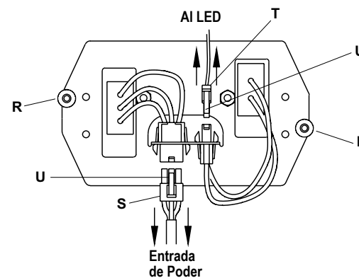
Figura 12b: Carcasas AX3(SQ) LPA/LPD
