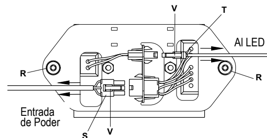
Figura 12b: Carcasas AX3(SQ) LPA/LPD
