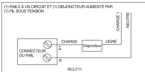
Schéma 2 (Alimentation en ligne)
