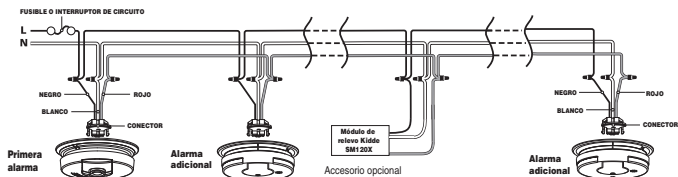
FIGURA 5 DIAGRAMA DE CABLEADO DE INTERCONEXIÓN
